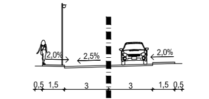
KARAKTERISTIČNI PRESJEK M1:200 PRESJEK A-A
